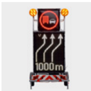
Remorque graphique à LED
